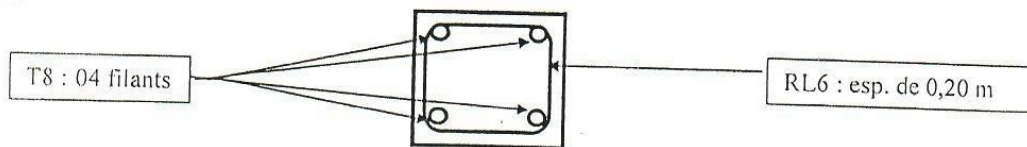
Coupe section poteau, poutre, linteau, longrine
